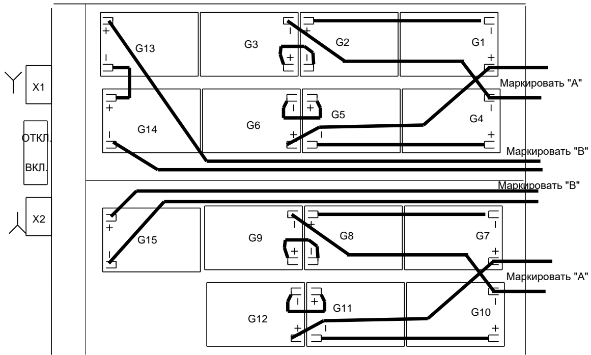
Рисунок 3 – Схема установки и соединений аккумуляторных батарей
